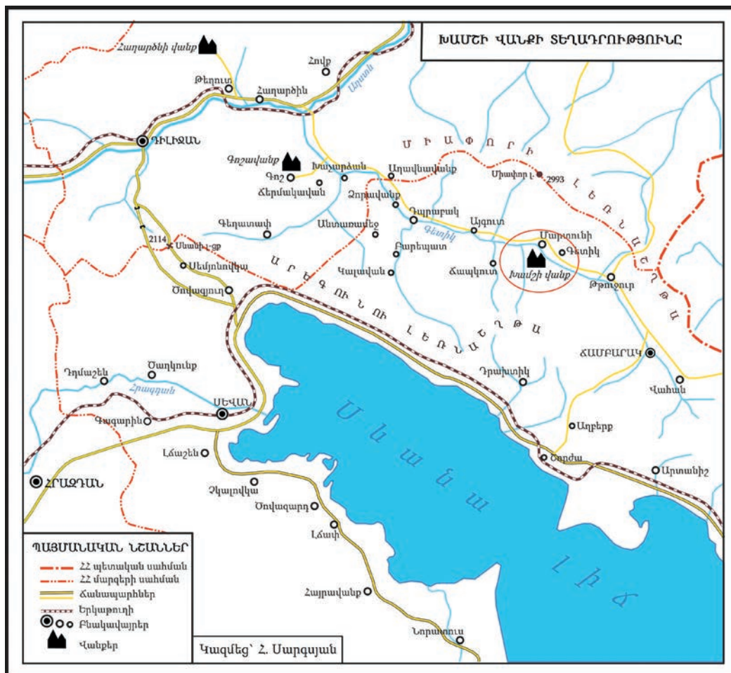
Քարտեզ 1. Խամշի վանքի տեղադրությունը (հեղ.՝ Հ. Սարգսյան, 2015 թ.)
